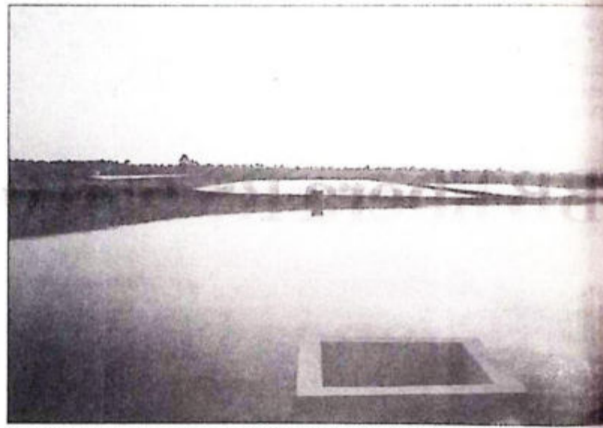
Lagoas de tratamento da Estação de Tratamento Sanitário de Trindade
