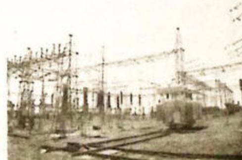
Subestação Anhangera (ampliação) Instalação de um transformador 138/69 KV, 25 mil KVA de potência
