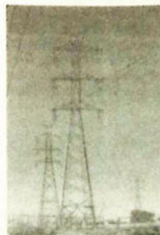
Linha de Transmissão Xavantes/Matinha (circuito duplo) 230 KV - 15,8 km
