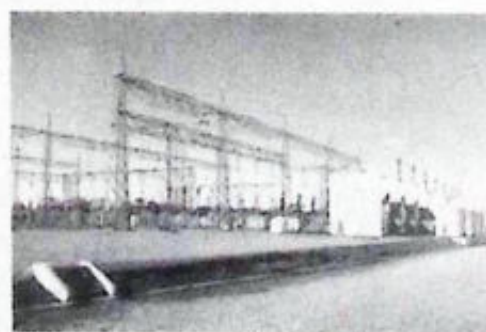
Subestação Xavantes (ampliação) Instalação do terceiro transformador 230/138 KV, 3 x 50 mil KVA de potência e 2 vias de linha de transmissão 230 KV para a interligação do sistema de Goiânia
