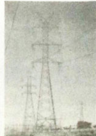
Linha de Transmissão Xavantes/Matinha (circuito duplo) 230 KV - 15,8 km
