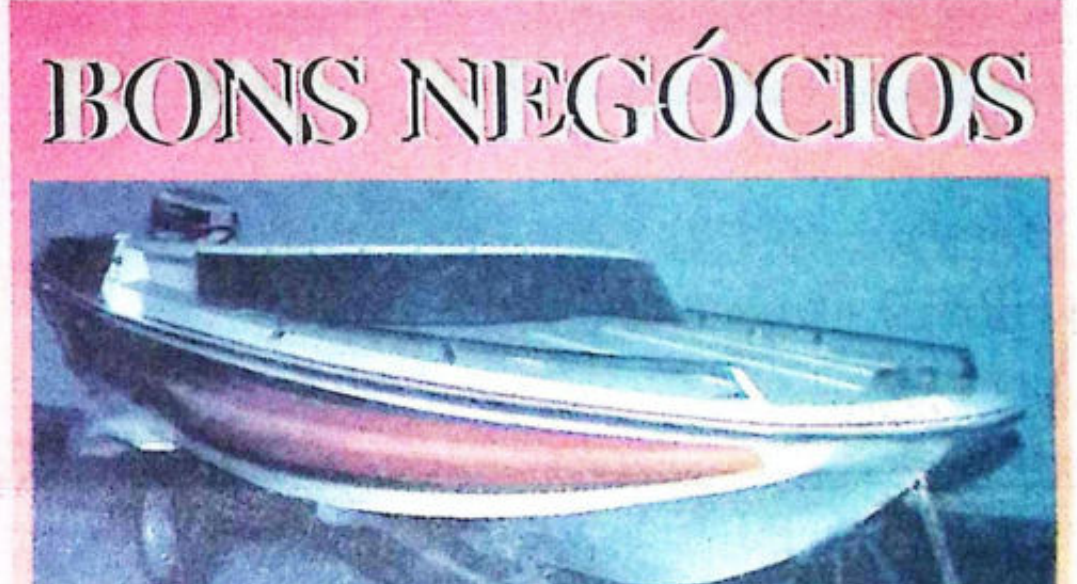
Vende-se esta lancha modelo Tranza, 16 pés, motor Johnson 60 HP, com bomba de porão. Tratar pelo fone 202-1806
