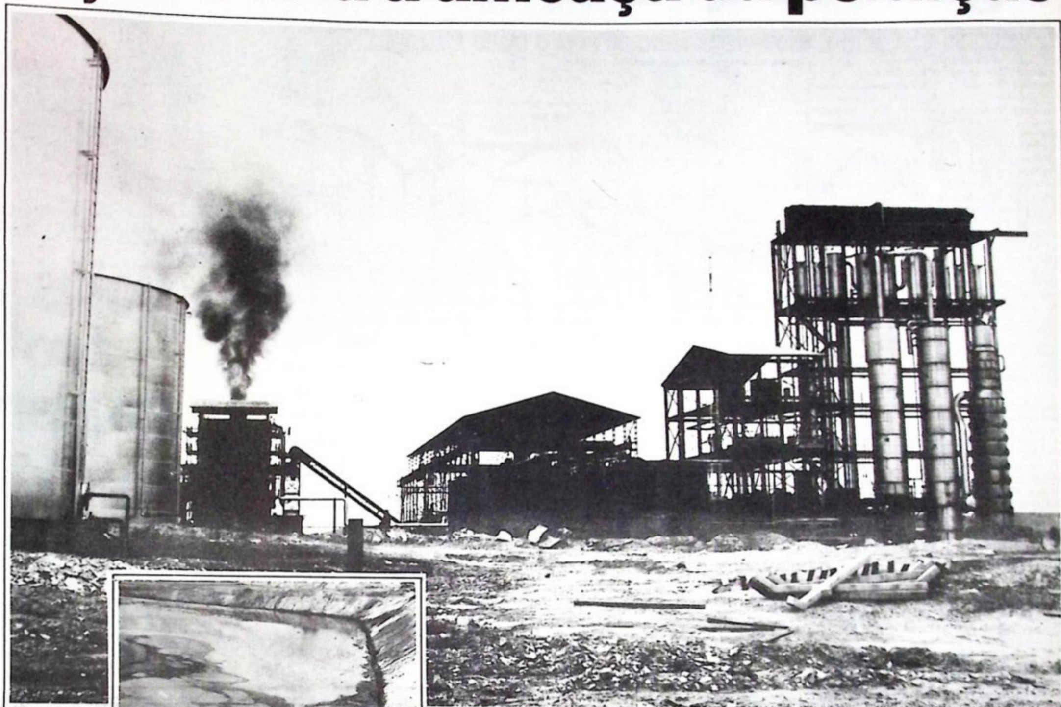
O bagaço é utilizado para aquecimento da caldeira e produção de energia elétrica
